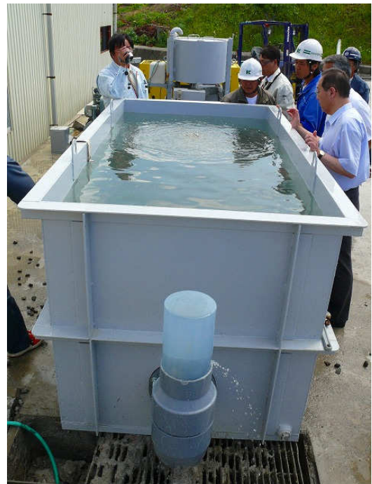
充填開始時の状況 吐出口から清水を排出
