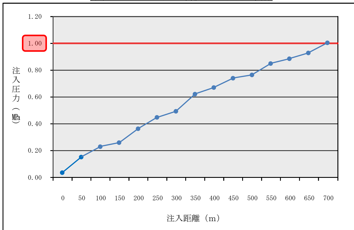
採取データ 圧送距離と注入圧力の関係
