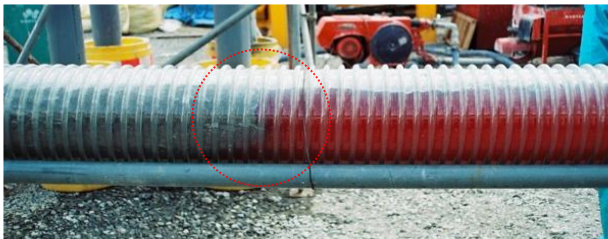
模擬施工での確認 満水状態の管内充填状況確認
