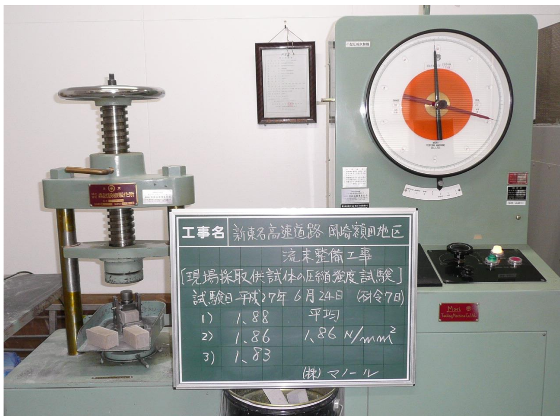
参考写真 小型強度試験機による圧縮強度試験
