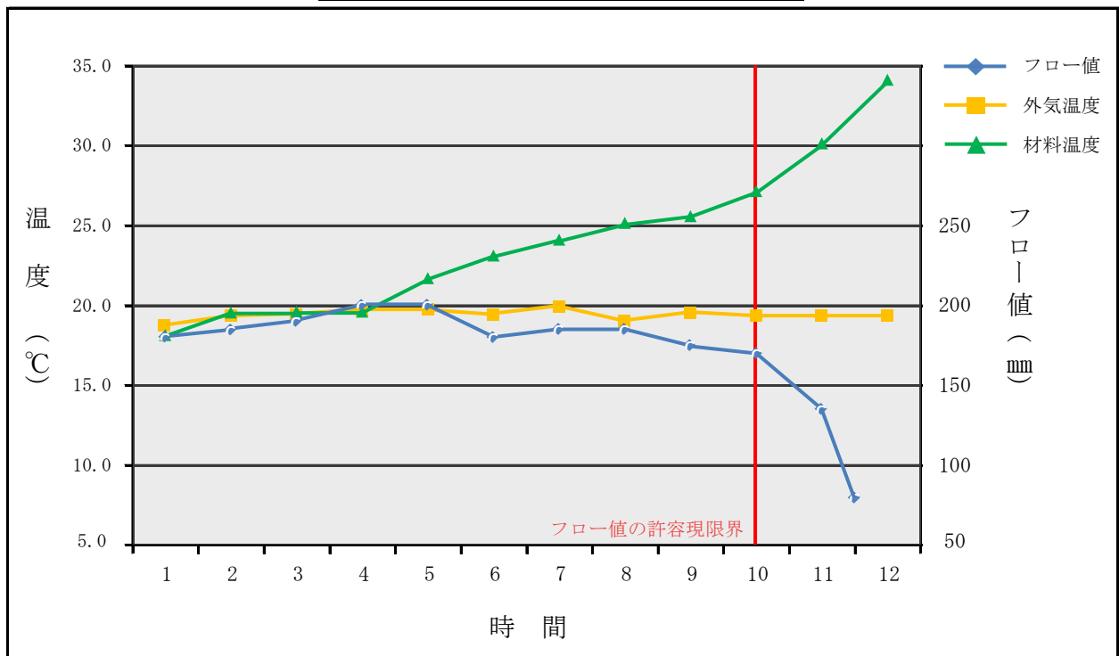
経過時間とフロー値・材料温度の関係
