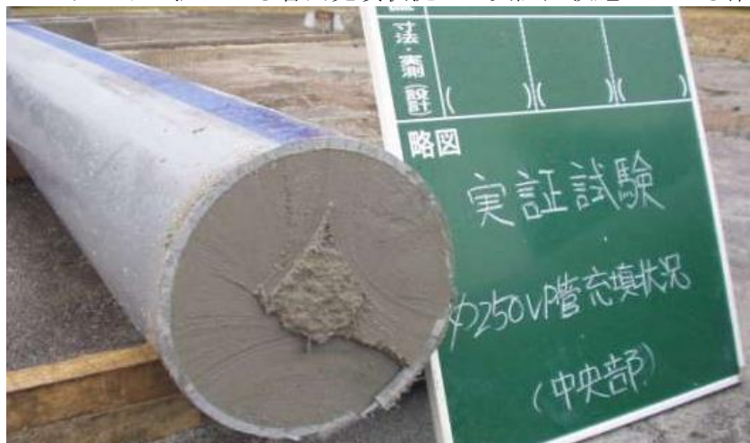
セルクリート工法による管内充填状況 実証試験施工による確認
