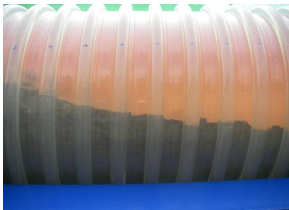
模擬施工での確認 満水状態の管内充填状況確認
